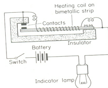
Fig. 15.7. Flasher unit
